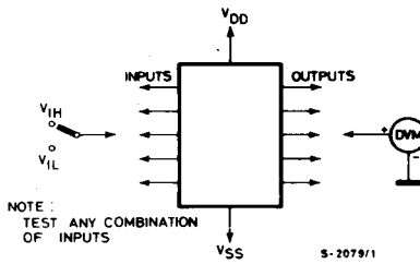
Input voltage
