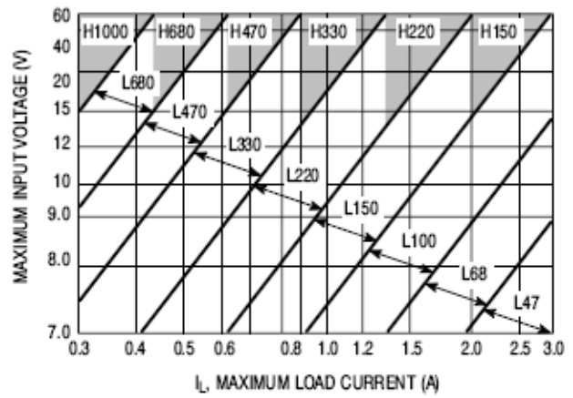
LM2576-5
