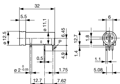
Variante 3101.0050
