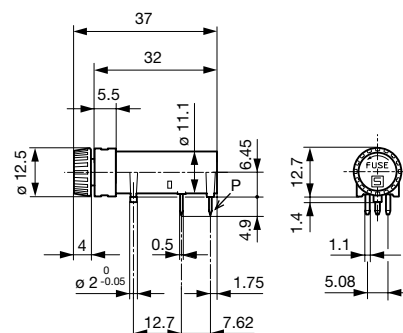
Variante Fingergrip 3101.0055
