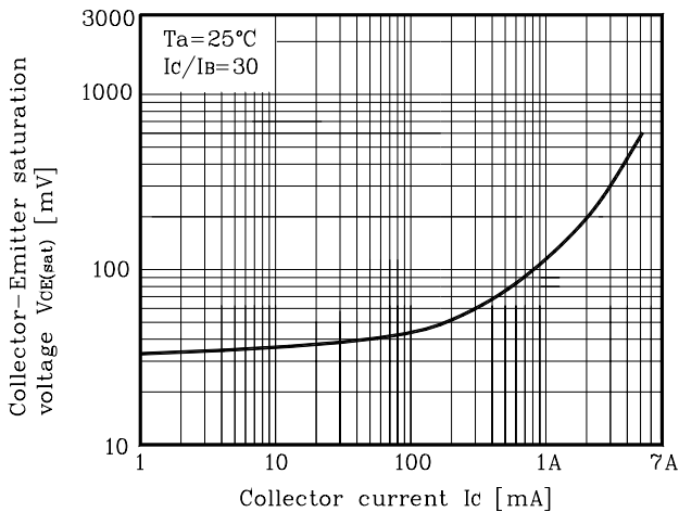
Fig. 3 V_{CE(sat)} - I_C
