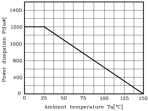
Fig. 1 P_c - T_a
