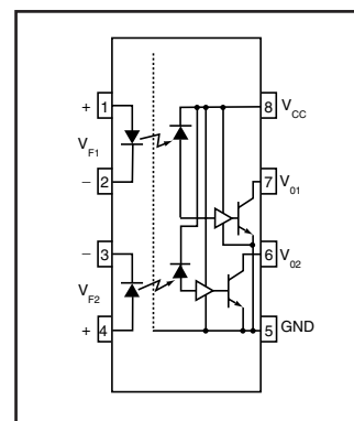
HCPL-2630 HCPL-2631
